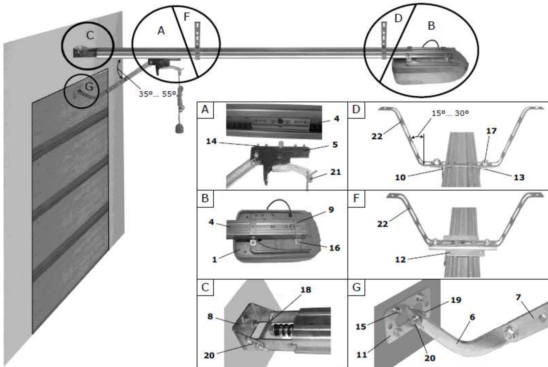
Рис. 2. Монтаж комплекта
